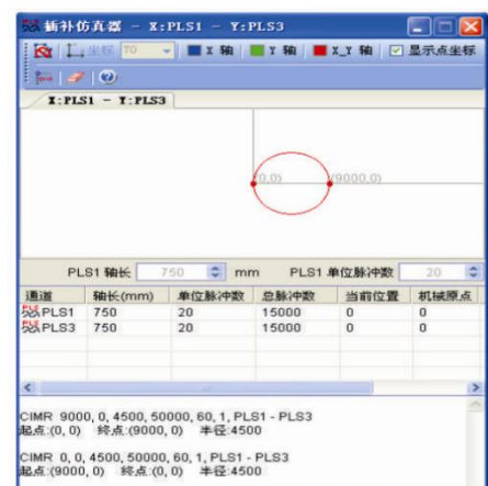
插补仿真器
